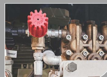
⑤ شیر تنظیم فشار Pressure Regulating Valve
