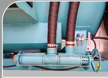
11 شیر چهار طرفه Four Way Valve
